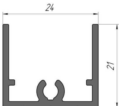
Профиль МП-3012
